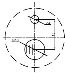
D部拡大
