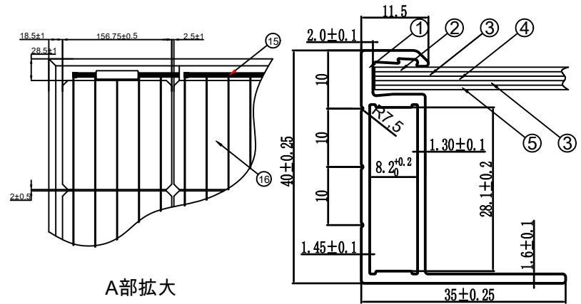
A-A'断面
