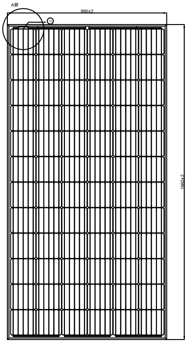
受光面
