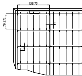
A部拡大
