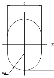
E部詳細
