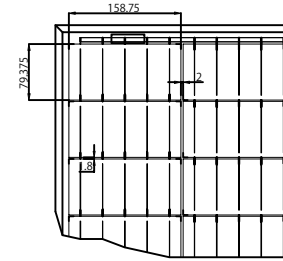
A部拡大
