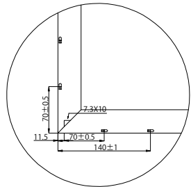
B部拡大
