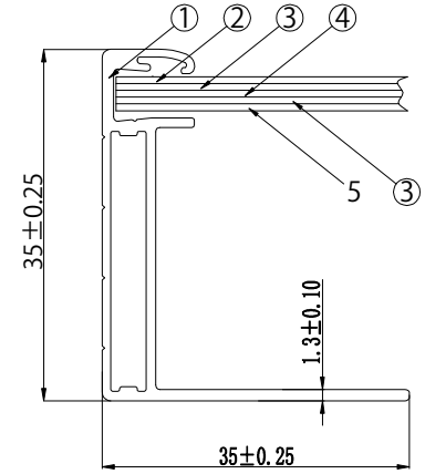
A-A'断面
