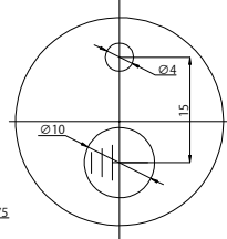
D部拡大
