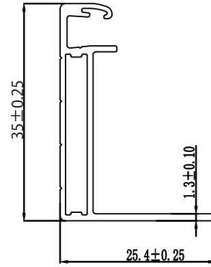
B-B'断面
