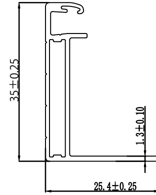
B-B'断面
