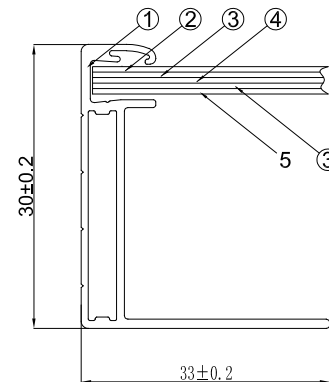
A-A'断面
