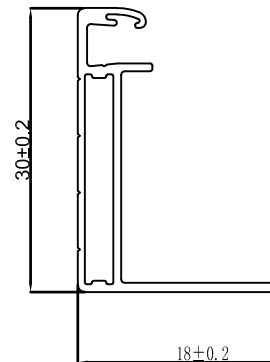
B-B'断面
