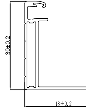
B-B'断面
