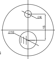
D部拡大
