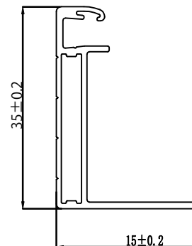
B-B'断面
