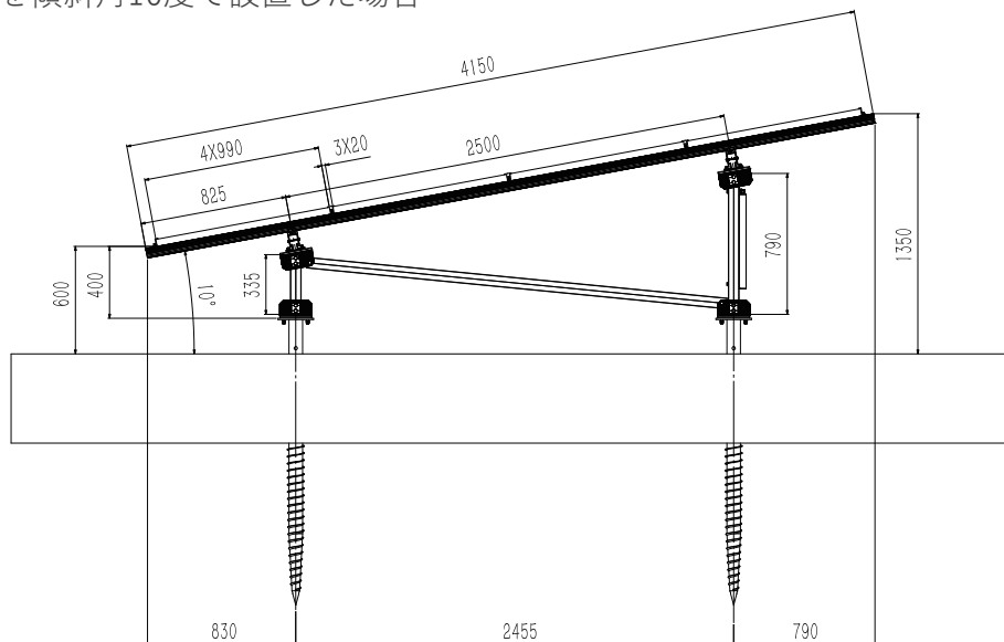
△側面
