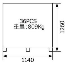
パレット単体: 36枚 パレット正面図
