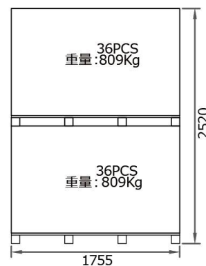
パレット2段: 72枚(36×2) 2段パレット側面図
