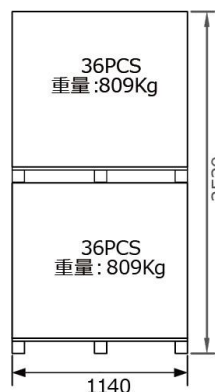
パレット2段: 72枚(36×2) 2段パレット正面図
