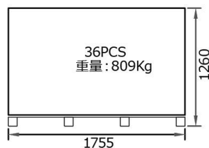
パレット単体: 36枚 側面図
