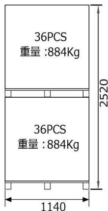
パレット2段：72枚(36×2) 2段パレット正面図
