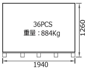
パレット単体：36枚 パレット側面図
