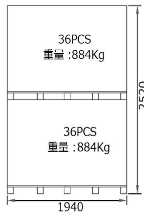
パレット2段：72枚(36×2) 2段パレット側面図
