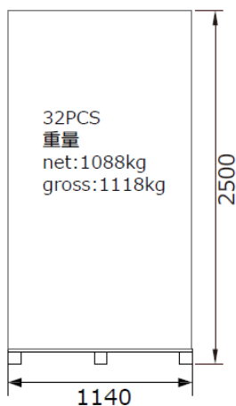
パレット単体：32枚 下段パレット正面図
