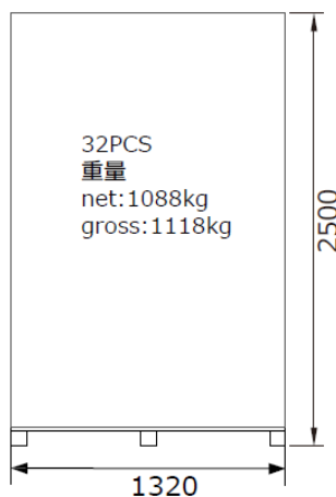
パレット単体：32枚 下段パレット側面図
