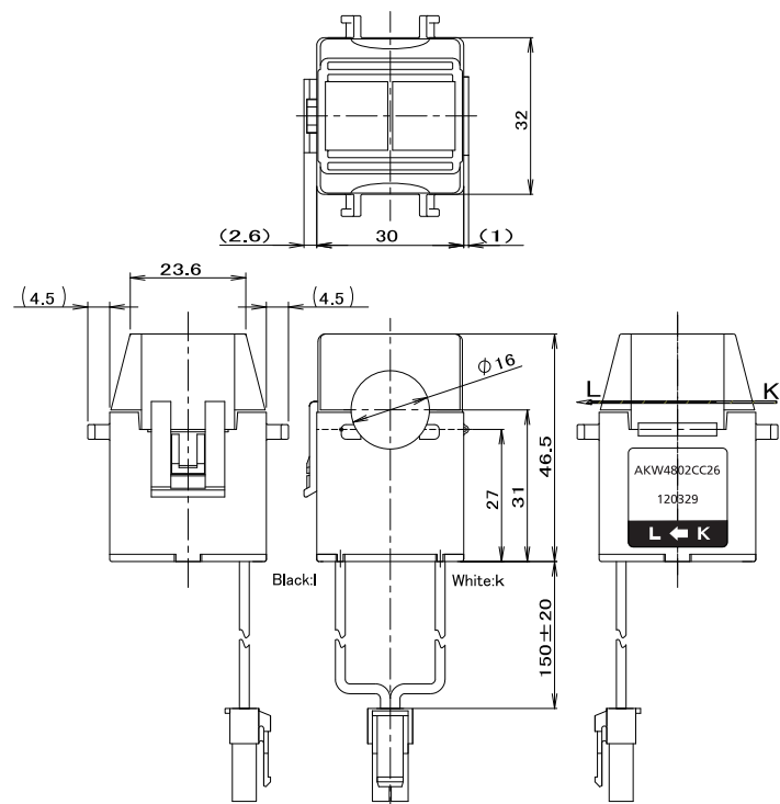
主幹電流センサ(内径16mm)
