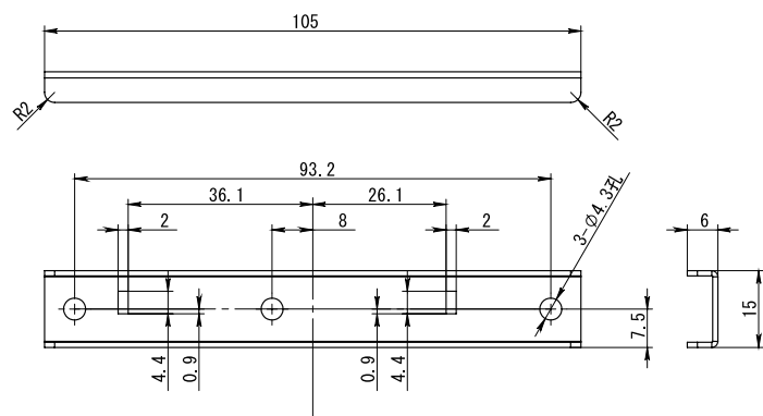
配線固定金具
