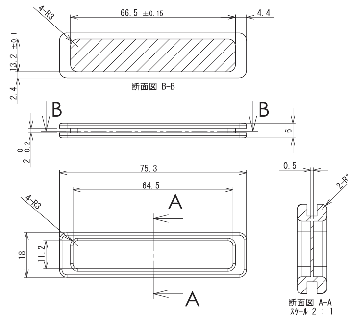
ブッシング
