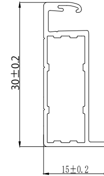
B-B'断面
