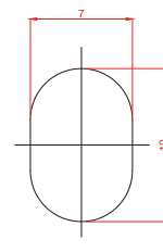
F部詳細
