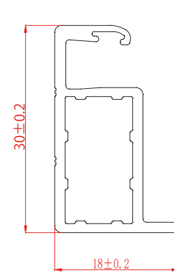
B-B'断面
