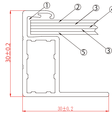
A-A'断面
