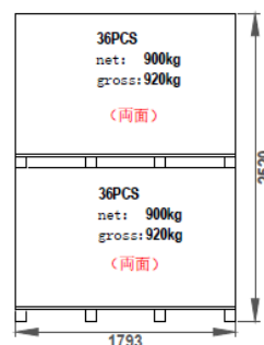
パレット合計:72枚 連結パレット側面図
