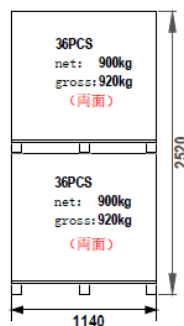
パレット合計:72枚 連結パレット正面図
