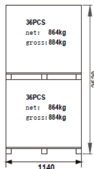
パレット単体：72枚 連結パレット正面図
