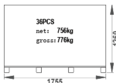
パレット単体：36枚 パレット側面図
