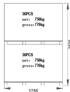
パレット単体：72枚 連結パレット側面図
