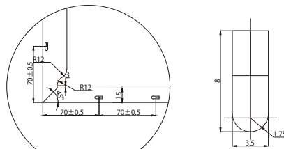
B部拡大
