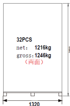
パレット単体：32枚 パレット側面図
