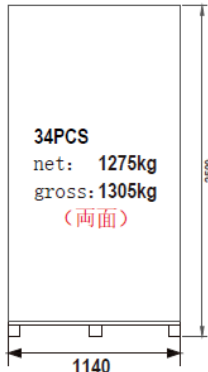
パレット単体：34枚 パレット正面図
