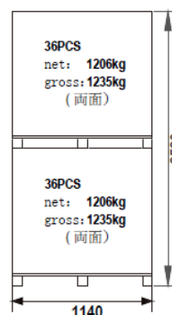
パレット合計：72枚 パレット正面図
