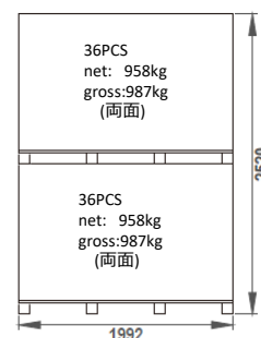
パレット合計：72枚 パレット側面図
