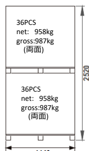
パレット合計：72枚 パレット正面図
