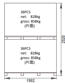
パレット合計：72枚 パレット側面図
