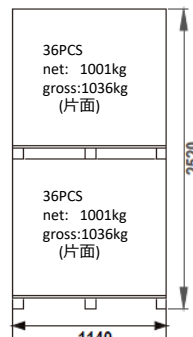
パレット合計：72枚 パレット正面図
