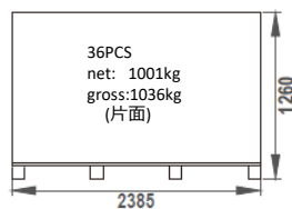
パレット単体：36枚 パレット側面図
