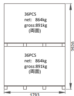
パレット合計：72枚 パレット側面図
