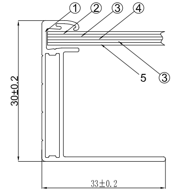
A-A'断面
