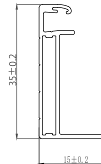
B-B'断面
