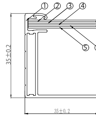
A-A'断面
