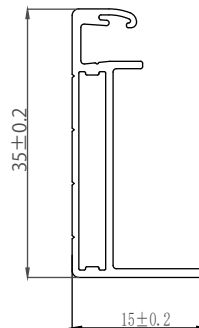
B-B'断面
